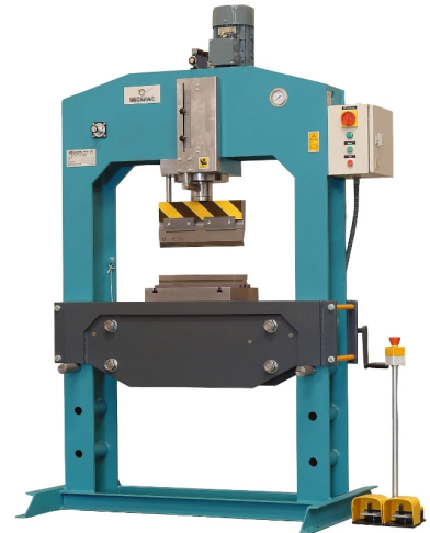
Prensa de 80 tm con opcional de equipo de plegado de 415 mm
